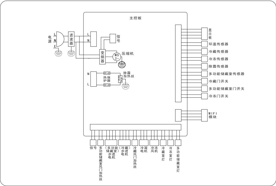
电路图（BCD-562WDGBTIWS）
